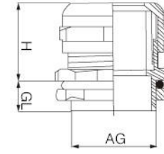
德制螺纹 PG 系列 PG thread type
